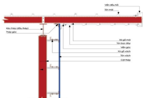
MÁI VƯỜN ĐẦU HỒI / ENDWALL WITH ROOF EXTENSION
