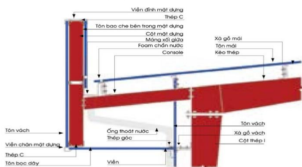
MẶT DỰNG ĐÚNG CỘ ĐÁY VÀ MĂNG XỐI FASCIA WITH SOFFIT AND VALLEY GUTTER
