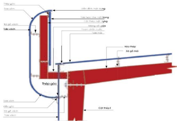
MẶT DỰNG CONG / CURVED FASCIA
