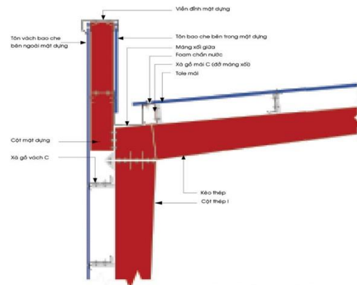
MẶT DỰNG TƯỜNG VƯỢT MÁI PARAPET FASCIA
