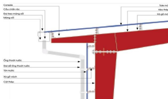
MÁI THẲNG TƯỜNG BIÊN / EAVE WITH ROOF EXTENSION
