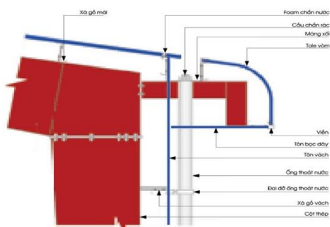
MÁI VƯỜN VỒM TƯỜNG BIÊN CURVED EAVE WITH VALLEY GUTTER AND SOFFIT
