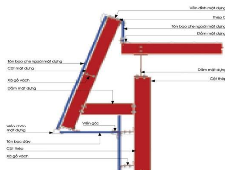
MẶT DỰNG NGHIÊNG / BEVEL FASCIA
